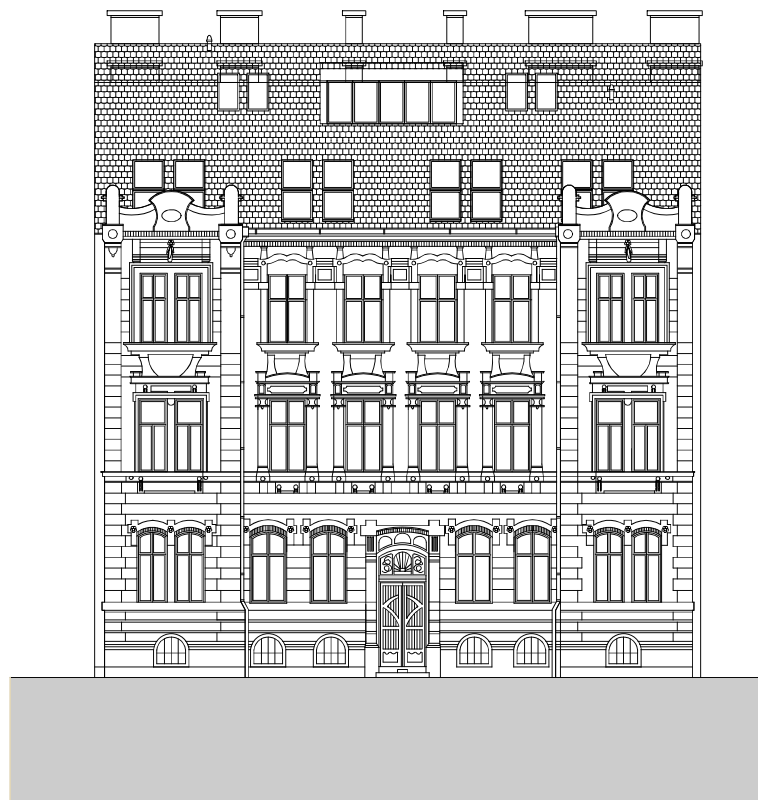
ULIČNÝ POHLAD
